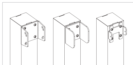
Soporte exterior para guía y perfil 100x120
