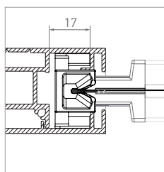
Sección guía ZIP
