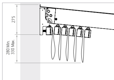
TX7910 PARED PORTERÍA
