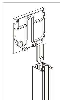
Detalle espiga tapa lateral y guía de 2 cuerpos
